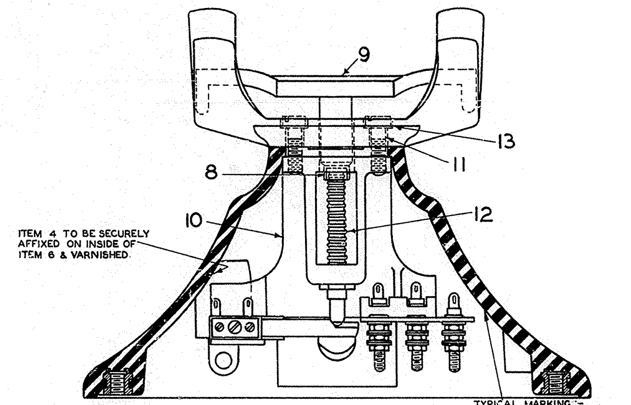
PART SECTION Y - Y (ITEM 5 OMITTED)
